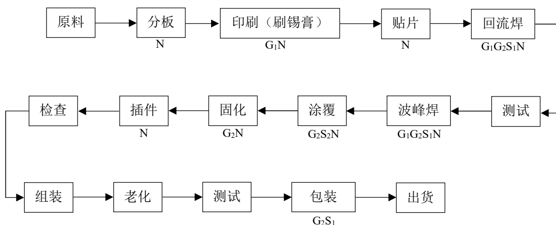
图 2-2 项目产品生产工艺流程图
